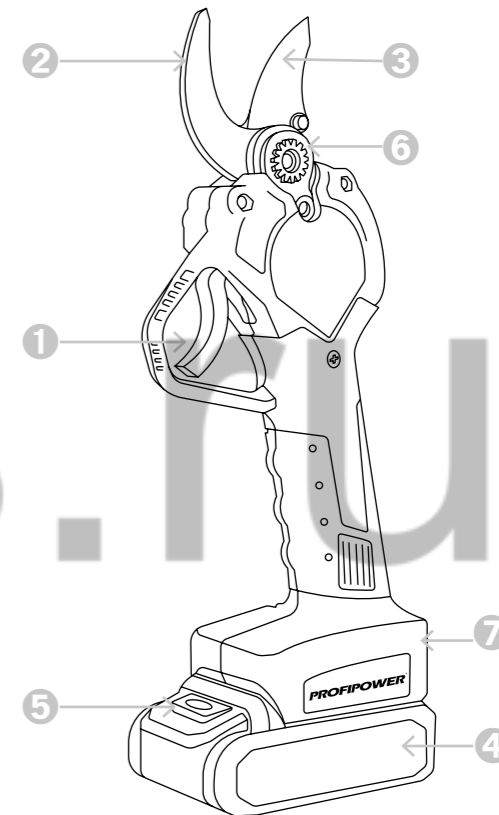
Рисунок 1.1. Устройство инструмента
